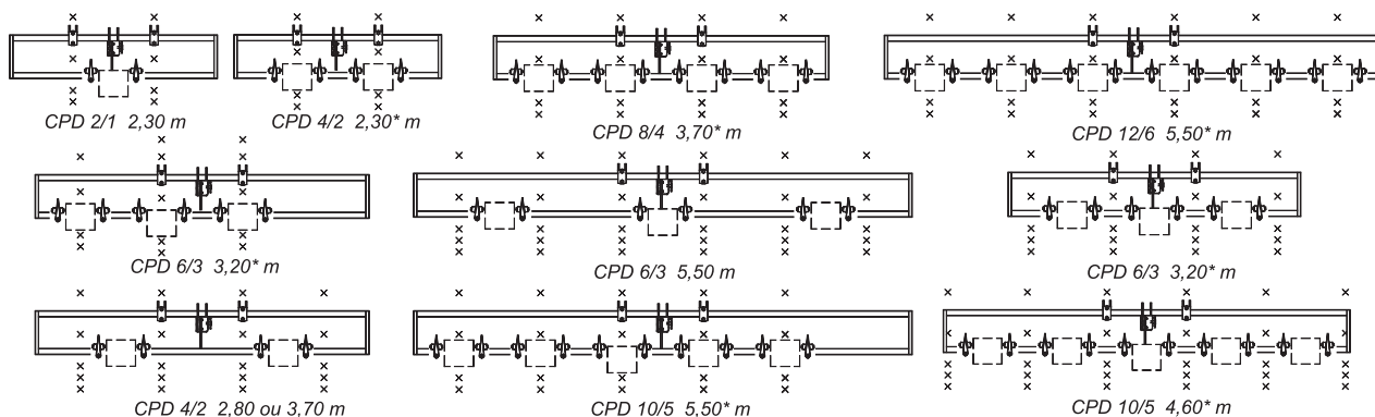
FRISOS LIMITADORES DE PROFUNDIDADE Ø 260 ou Ø 280 mm acoplados aos discos duplos.
