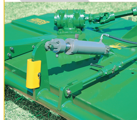
Regulador da altura de corte no cilindro. Varão estabilizador para nivelamento da roçadeira.
