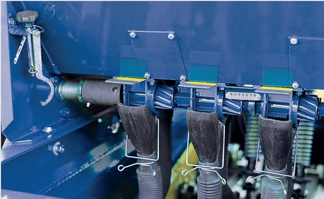
Rotores acanalados helicoidais com fácil ajuste para diferentes tipos e quantidades de sementes.
