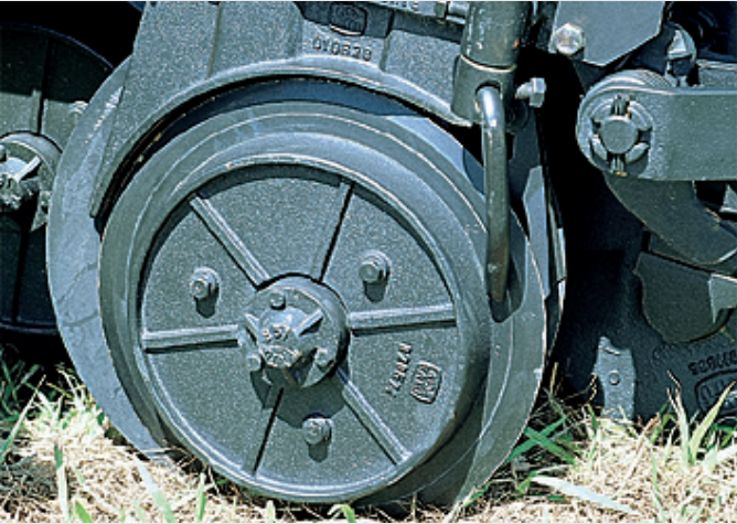
FRISOS LIMITADORES DE PROFUNDIDADE Ø 310 ou 330 mm
