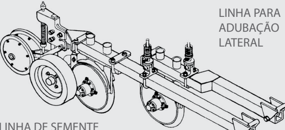
LINHA DE SEMENTE PARA SOJA
