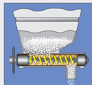
Distribuição de adubo através de Condutores Helicoidais (Sem-Fim). Com revestimento interno de PVC. Maior uniformidade no plantio.
