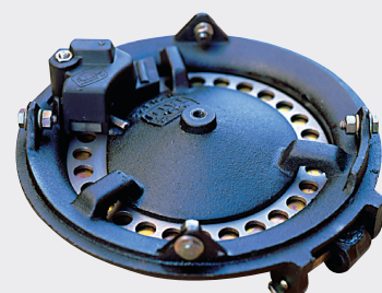
Discos horizontais perfurados para diferentes culturas e tamanhos de grãos. Discos de semente fornecidos por linha: 01 para milho, 01 para soja e 01 cego.
